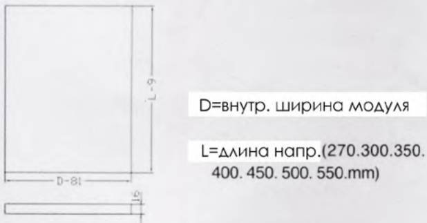
Размеры днища ящика (для 16 мм ДСП)
